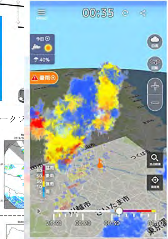
PAWR Obs
