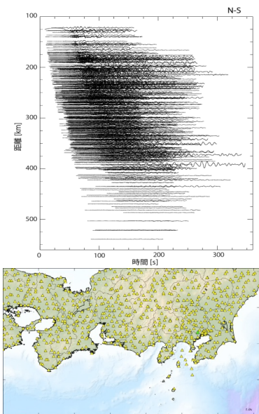
90秒間の同化→予測計算
