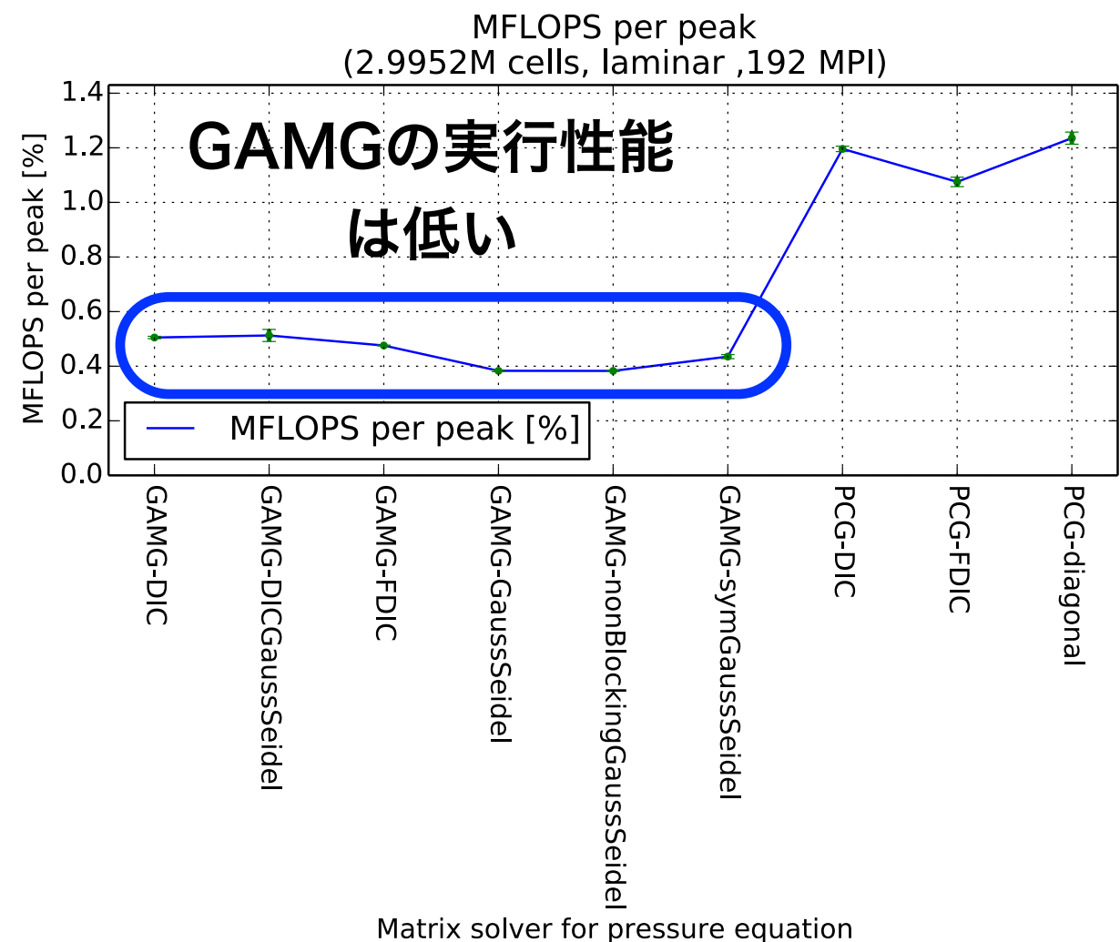
圧力線型ソルバと実行性能の関係 (192MPI並列)
