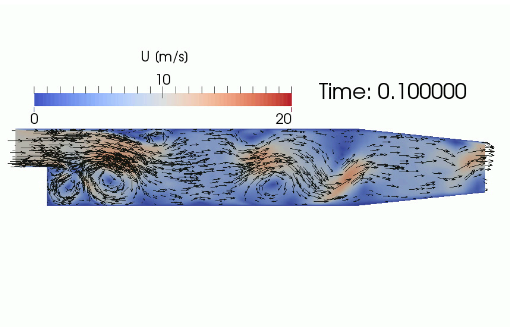
バックステップ流れ pitzDaily
