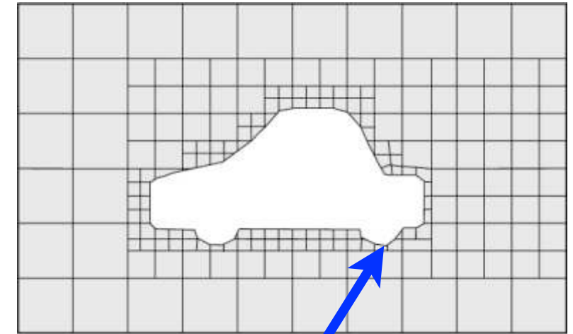
境界適合
