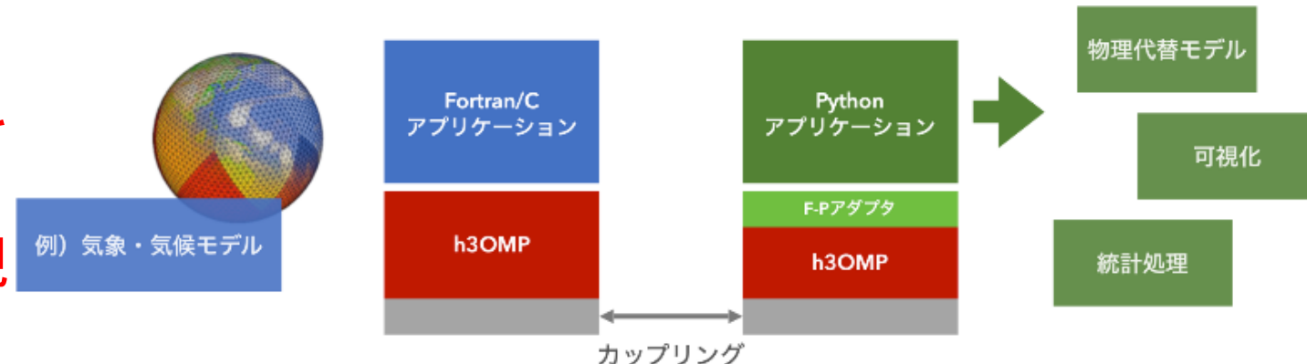
Fortran/CアプリとPythonアプリの連成計算の模式図 〔八代・荒川 2020〕
