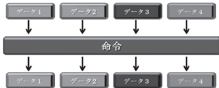
図 2 SIMD の概念
